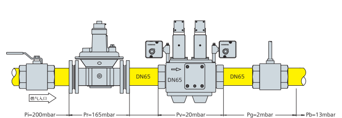
阀前减压压差分布图：
